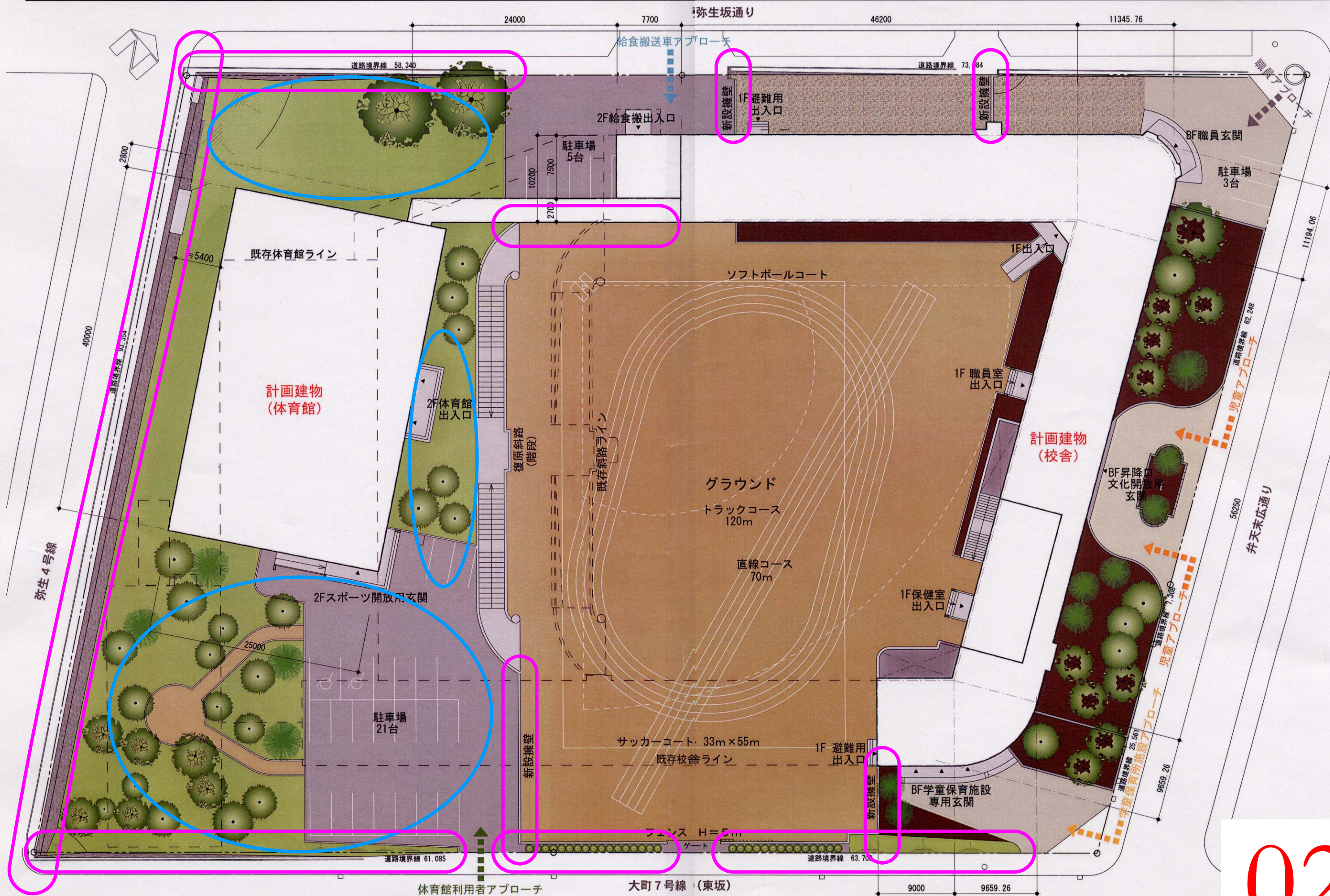
配置・外構図 S3=1:400
